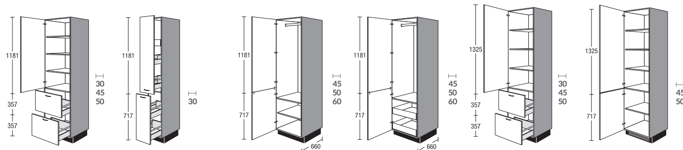
S2A... 01 Armoire Hoge kast
