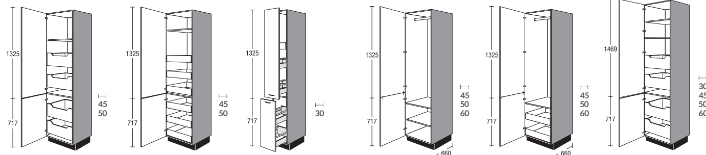
S... 02 IA Armoire Hoge kast
