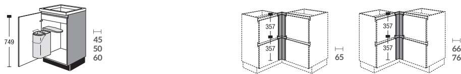
CSP...MT1 Meuble bas sous-évier Spoelkast CUPEF...M2 Fileur d'angle pour meubles bas Hoekpaslijst voor onderkasten CUPEF...VM2 Fileur d'angle pour meubles bas Hoekpaslijst voor onderkasten CUPEF...VGS2 Fileur d'angle pour meubles bas Hoekpaslijst voor onderkasten
