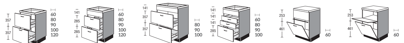
KD2A...U Meuble bas pour table de cuisson avec aérateur de plan de travail Kookplaatkast voor werkbladafzuiging KDB2A...U Meuble bas pour table de cuisson avec aérateur de plan de travail Kookplaatkast voor werkbladafzuiging KDB2A...87 U Meuble bas pour table de cuisson avec aérateur de plan de travail Kookplaatkast voor werkbladafzuiging KDB2SA...U Meuble bas pour table de cuisson avec aérateur de plan de travail Kookplaatkast voor werkbladafzuiging SPBG... Meuble bas sous-évier pour lave-vaisselle compact Spoelkast voor compacte vaatwassers SPKG... Meuble bas sous-évier pour lave-vaisselle compact Spoelkast voor compacte vaatwassers
