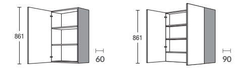
CHD...03 Meuble suspendu pour hotte cache-lumière Bovenkast voor lichtlijst-afzuigkap CHD...03 Meuble suspendu pour hotte cache-lumière Bovenkast voor lichtlijst-afzuigkap
