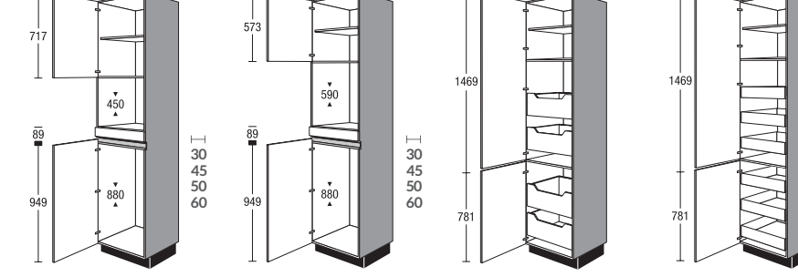
CG88M 03 H4 Armoire Hoge kast
