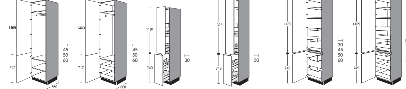
S... 03 66G1 Armoire avec tringle à habits Hoge kast met kledingstang
