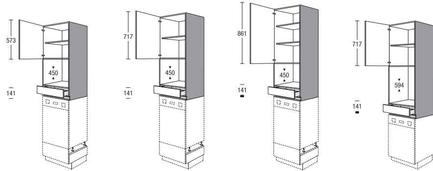
CAMS 124 H Demi-armoire Opzetkast
